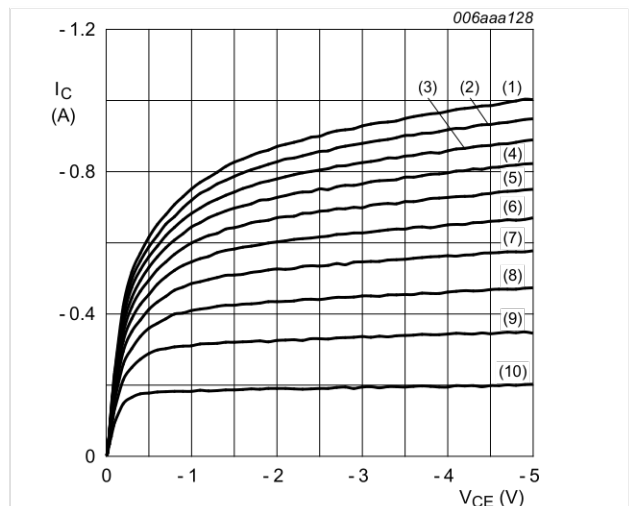
T_{amb} = 25\text{ °C} (1) I_B = -16.0\text{ mA} (2) I_B = -14.4\text{ mA} (3) I_B = -12.8\text{ mA} (4) I_B = -11.2\text{ mA} (5) I_B = -9.6\text{ mA} (6) I_B = -8.0\text{ mA} (7) I_B = -6.4\text{ mA} (8) I_B = -4.8\text{ mA} (9) I_B = -3.2\text{ mA} (10) I_B = -1.6\text{ mA}
