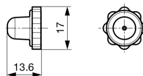
Schutzabdeckung TZZ31 für IP65 optional, siehe Zubehör
