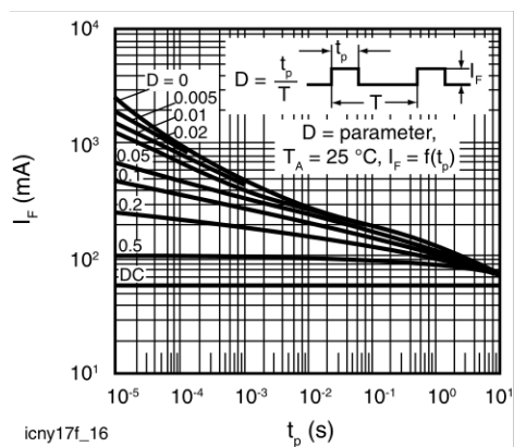
Fig. 16 - Permissible Pulse Load
